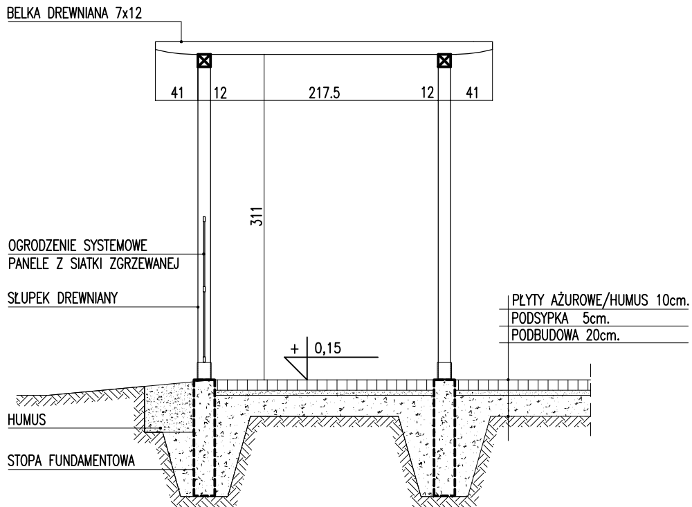
PRZEKRÓJ POPRZECZNY
