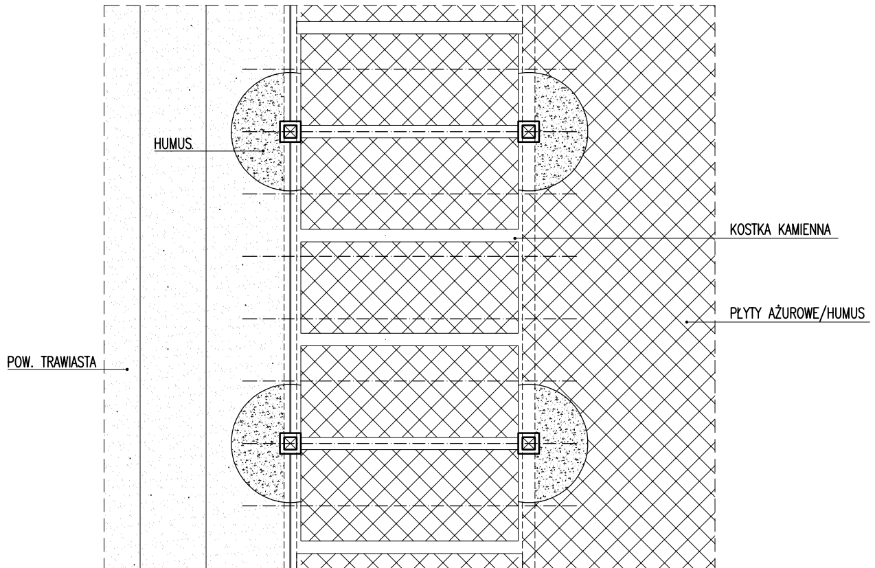
FRAGMENT RZUTU
