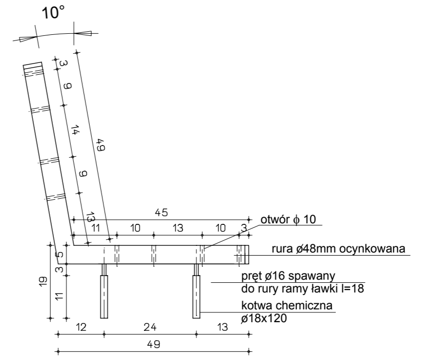
Detal "A", skala 1:10
