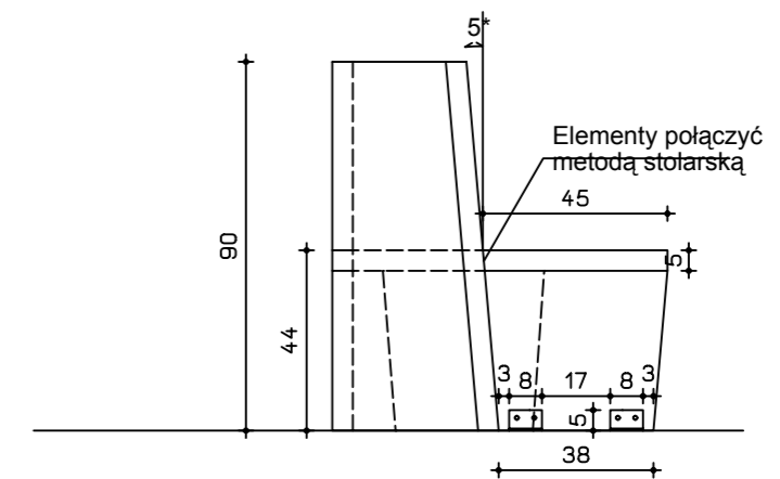
PRZEKRÓJ H-H
